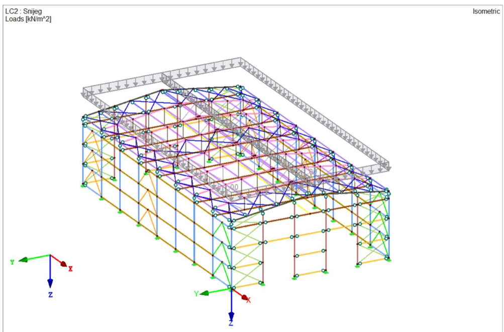
Slika 4.3.2.: Opterećenje snijegom
