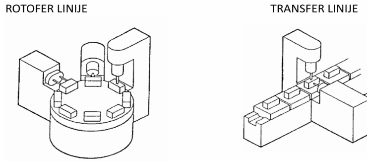
Slika 19. Primjer rotofer i transfer glodaće linije [13]
