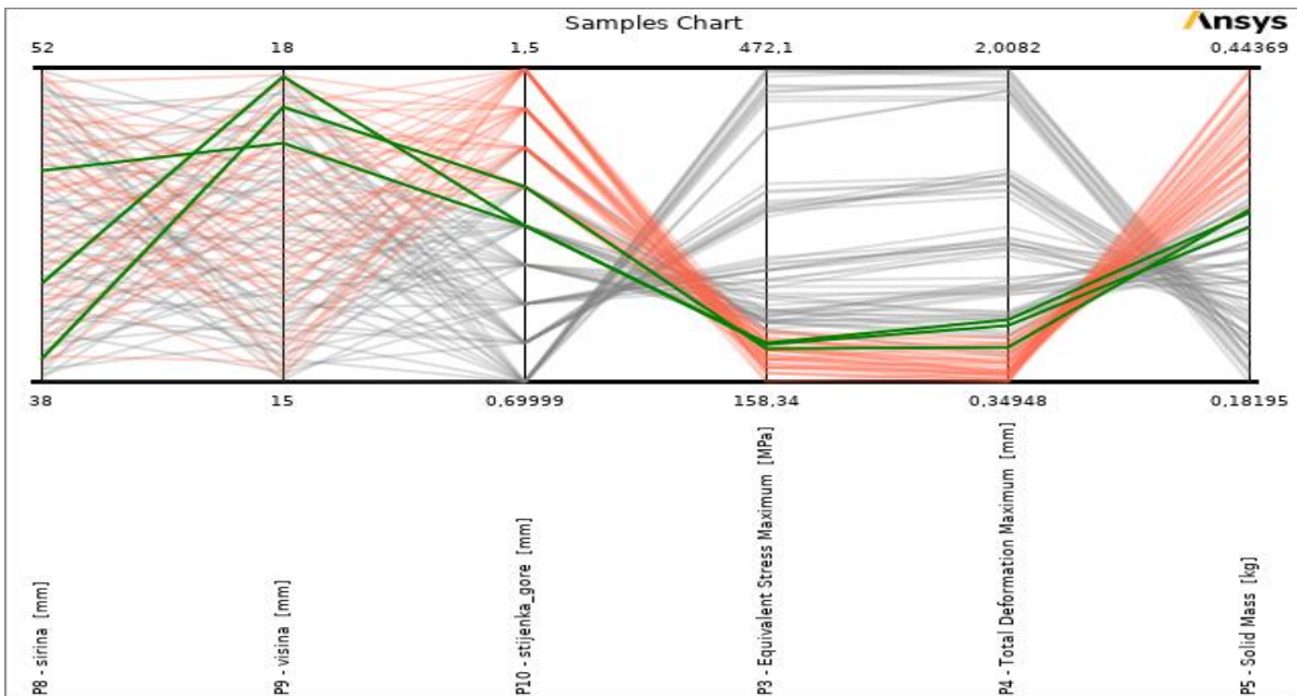
Slika 4.14 Najbolji kandidati optimizacije prečke
