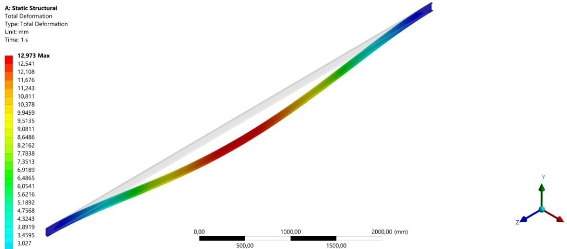
Slika 3.19 Simulacija šine (a ekvivalentan von Misesova napreznja (b progib
