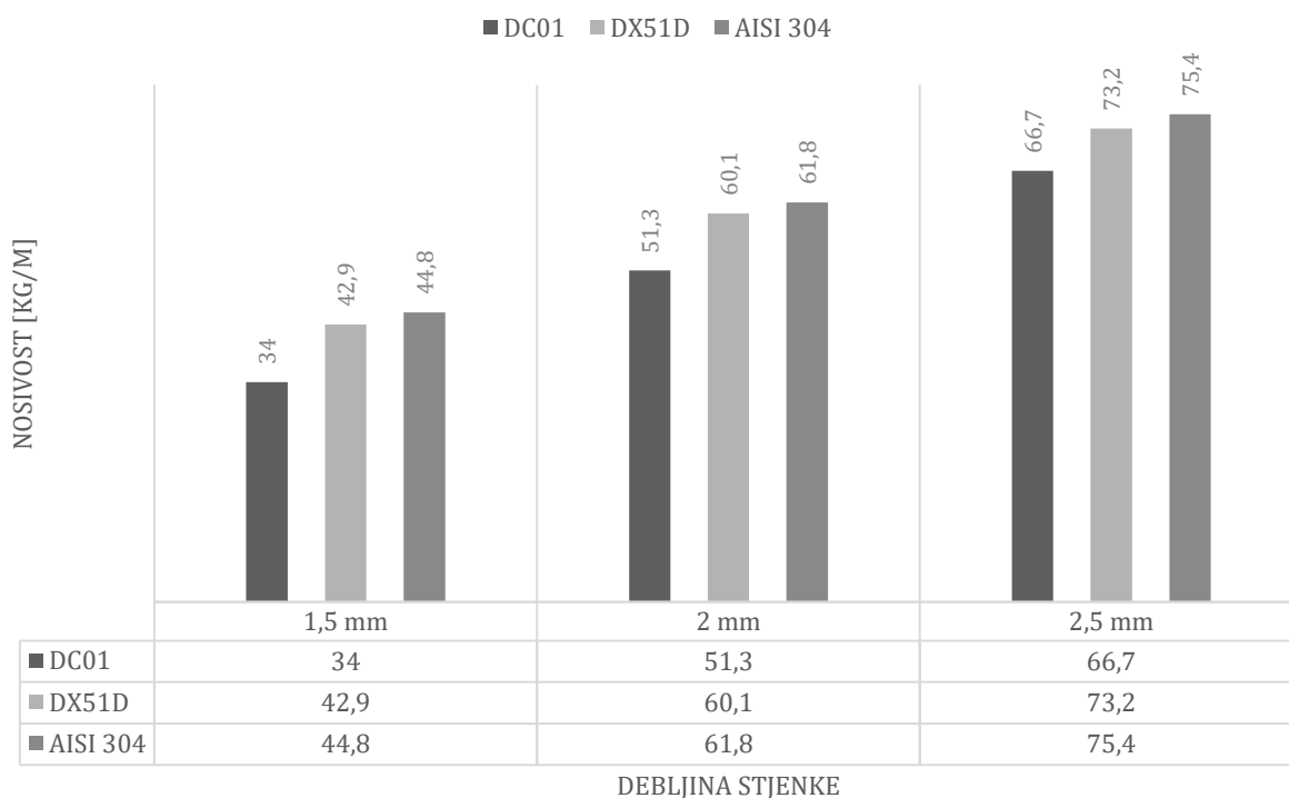
Graf 3.6 Utjecaj debljine stjenke kabljskih ljestava na nosivost
