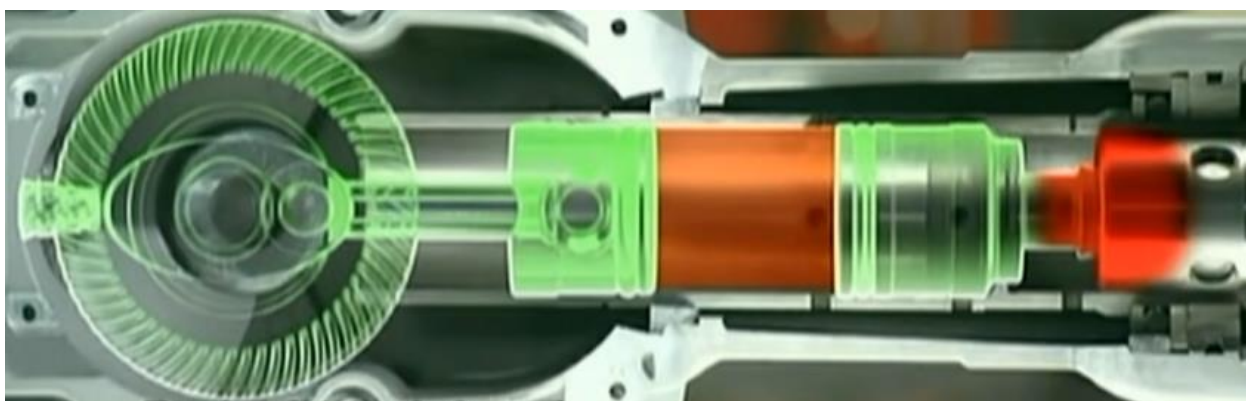
Slika 3. Prikaz kretanja klipa naprijed [33]
