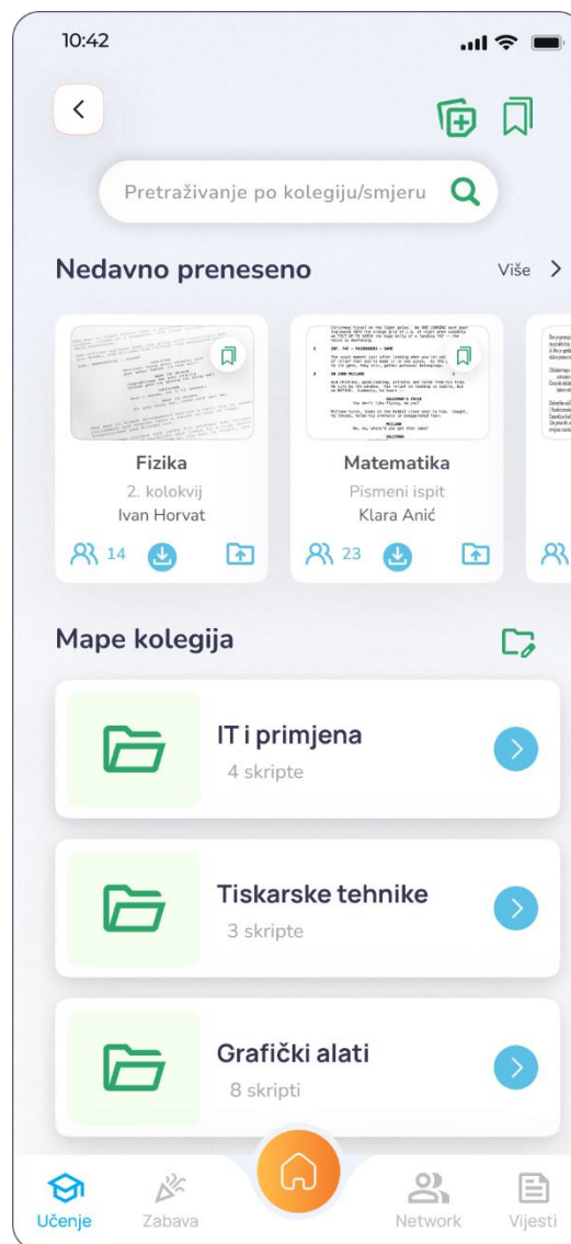
Slika 9.12 Skripte
