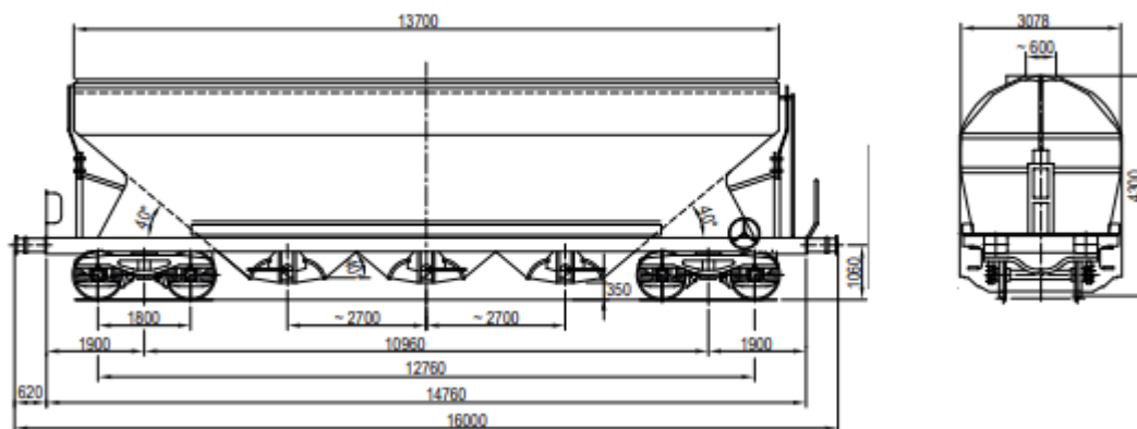
Slika 13. nacrt VTG tagnpps vagona H45.102D
