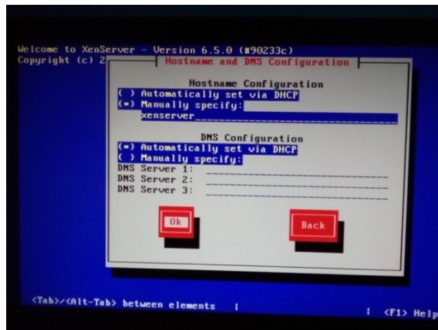
Slika 42: XenServer - instalacija (5)
