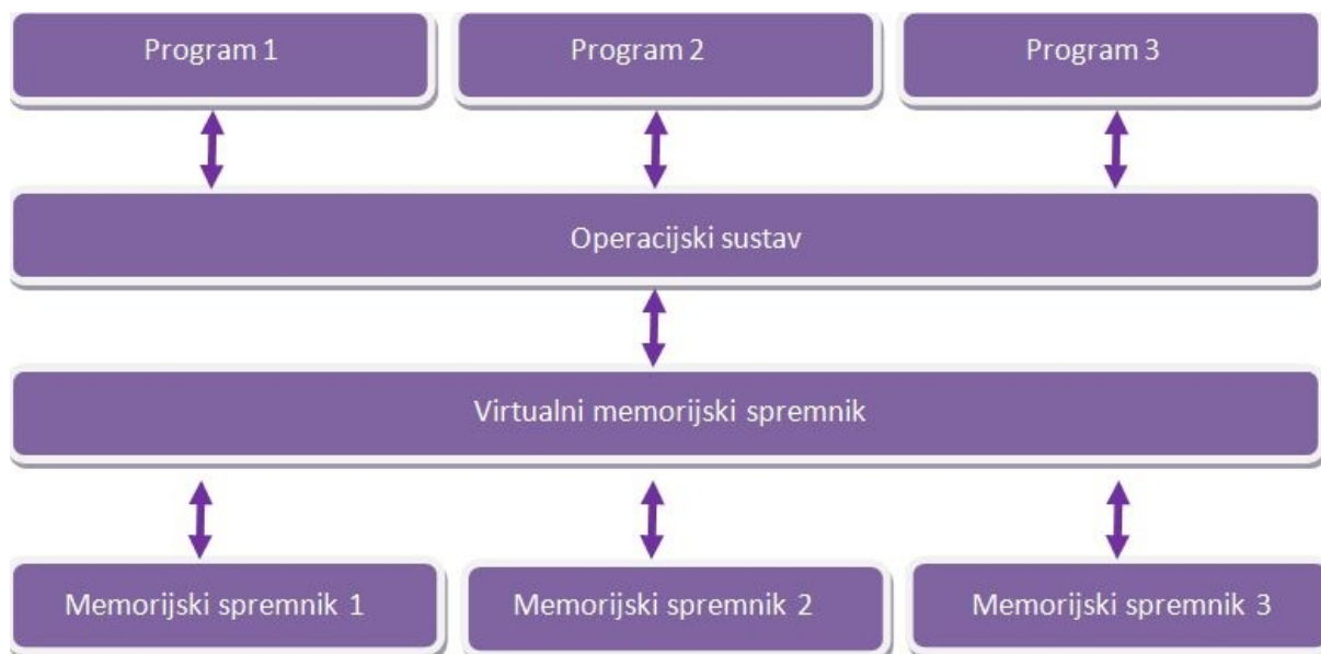
Slika 4: Virtualizacija memorije [3]
