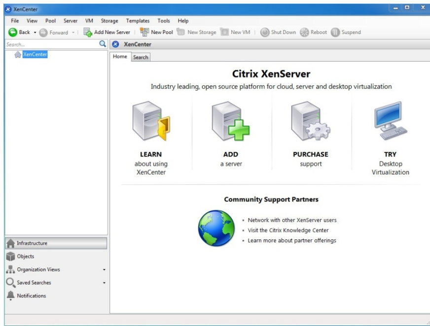
Slika 44: XenCenter
