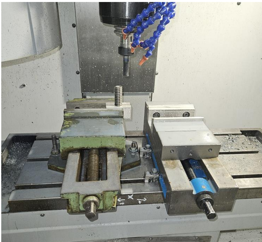
Slika 35: Glodanje šesterokuta na trapeznom navoju[osobne slike]
