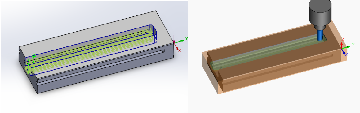
Slika 29: Putanje alata i simulacija kod glodanja srednjeg utora - 2. stezanje [osobne slike]
