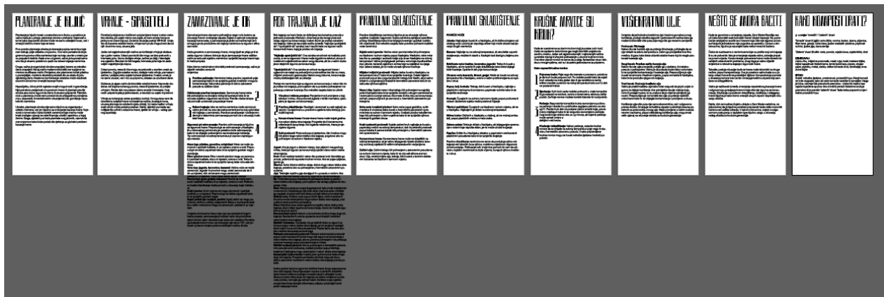
Slika 5.9 Postava teksta
