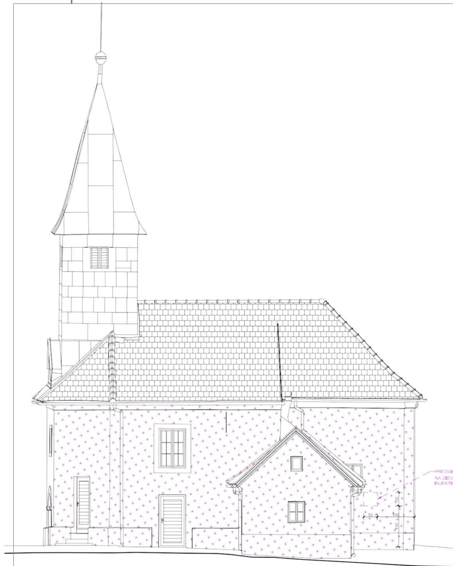
JUŽNO PROČELJE
