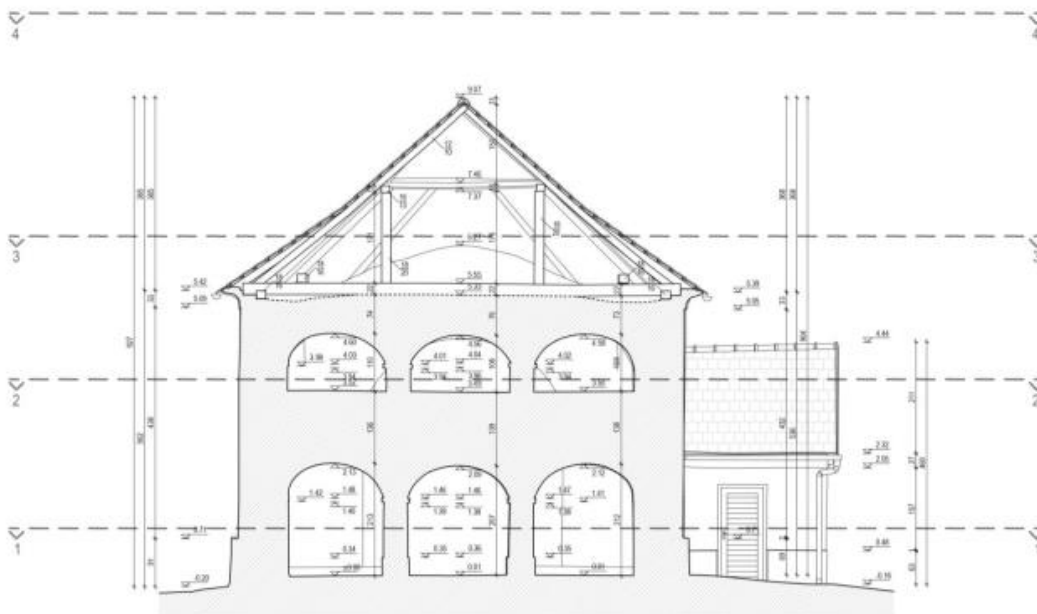
Slika 26: Presjek 3-3 [4]
