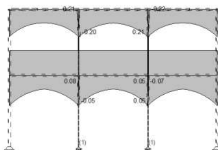
Okvir: V_6 Utjecaji u gredi: max M1= 0.21 / min M1= -0.22 kNm
