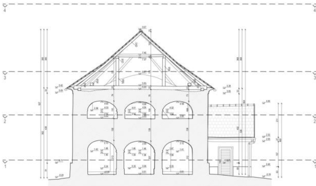
Slika 26: Presjek 3-3 [4]
