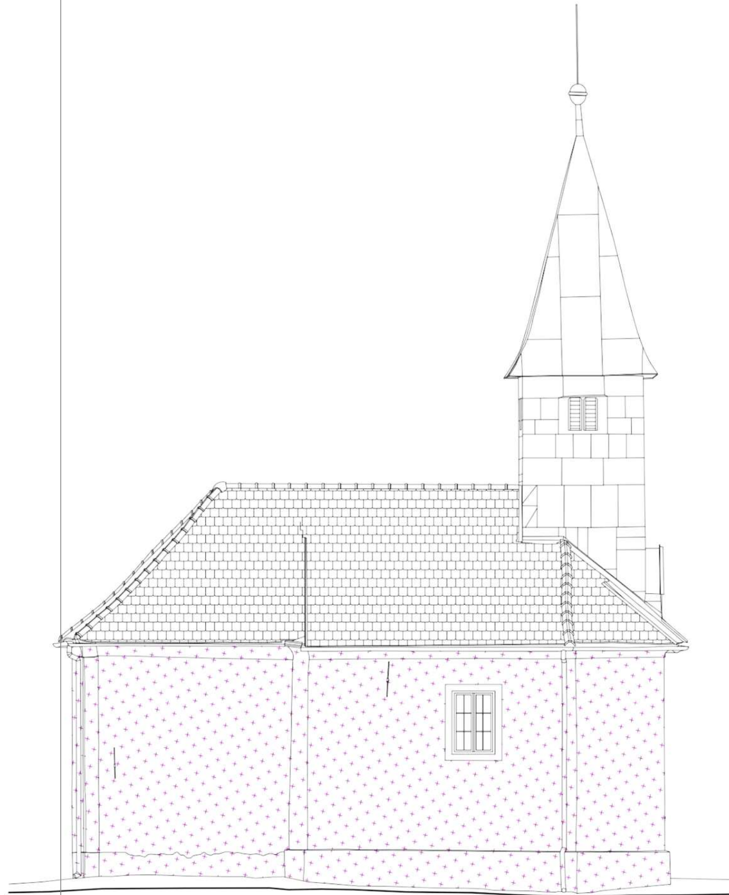
SJEVERNO PROČELJE
