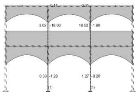
Okvir: V_6 Utjecaji u gredi: max T3= 18.52 / min T3= -18.06 kN
