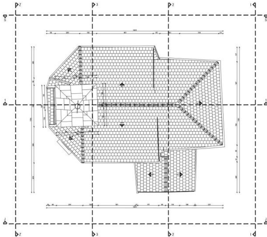
Slika 23: Tlocrt – razina 5 [4]
