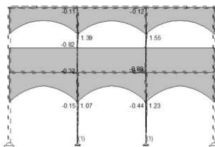
Okvir: V_6 Utjecaji u gredi: max M3= 1.55 / min M3= -0.89 kNm
