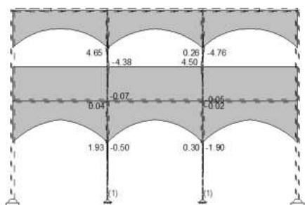
Okvir: V_6 Utjecaji u gredi: max M2= 4.65 / min M2= -4.76 kNm
