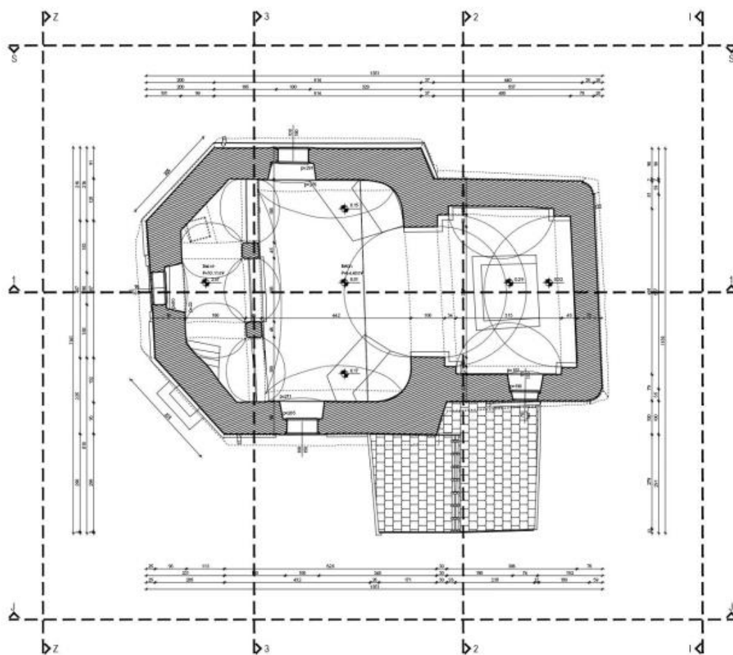
Slika 20: Tlocrt – razina 2 [4]
