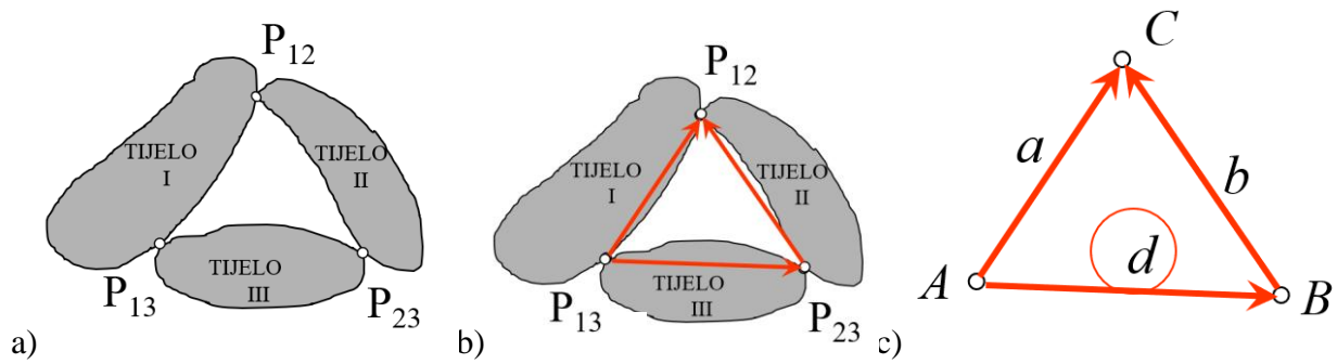
Slika 2.4 Dokaz Kennedyevog teorema
