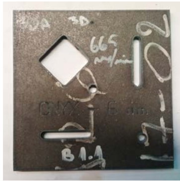
Slika 4.3.18. Uzorak B4.1 debljine 6 mm s podacima o rezanju
