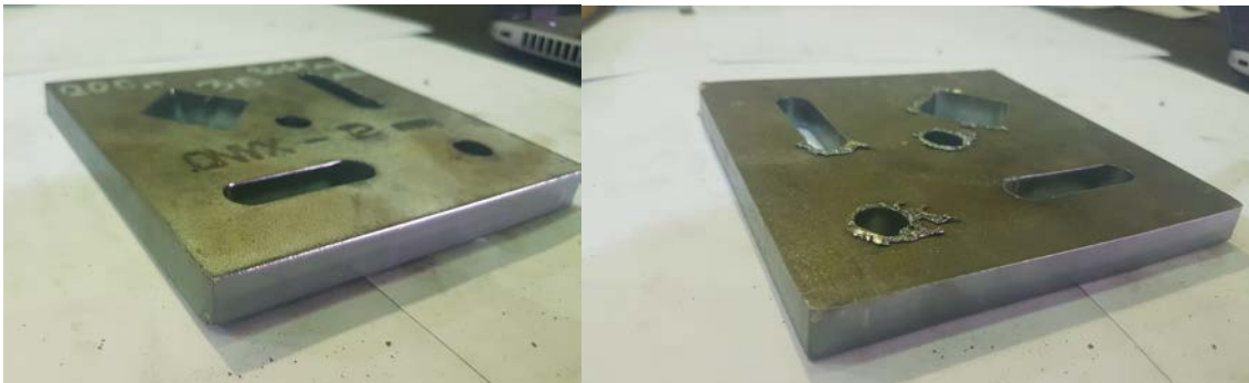
Slika 4.3.35. Uzorak B7.2 debljine 12 mm slikan s gornje i donje strane
