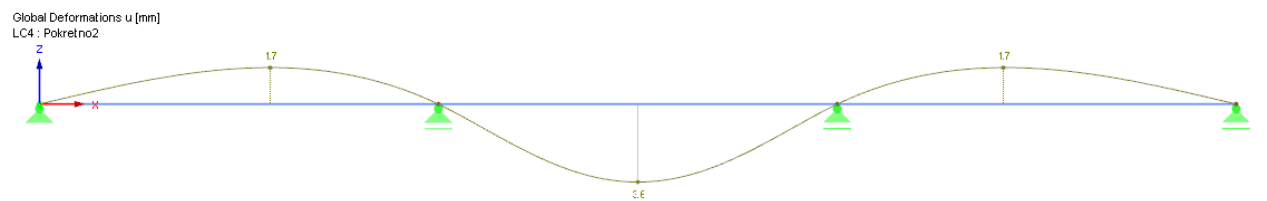
Slika 67 Deformacije [mm]
