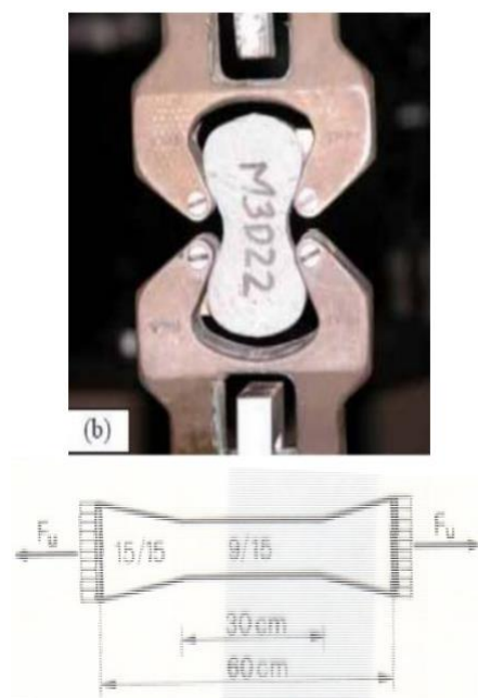
Slika 12. Ispitivanje vlačne čvrstoće
