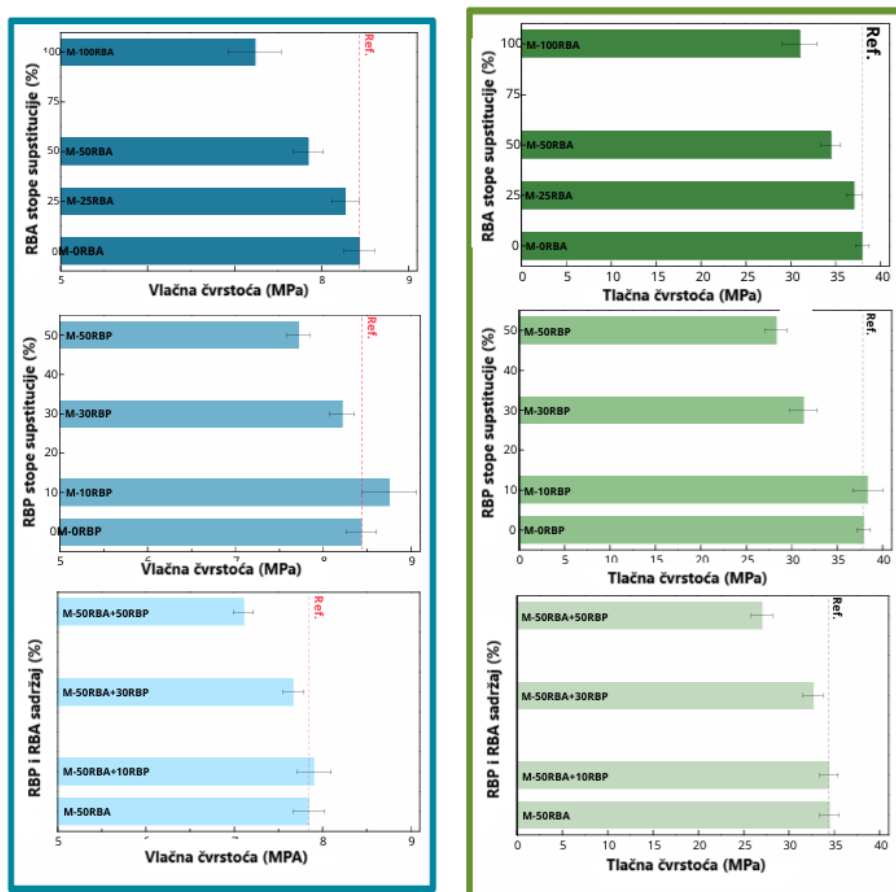
Slika 34. Vlačna i tlačna čvrstoća cementog morta s RBP i RBA [13]
