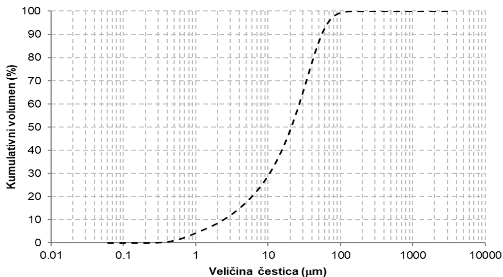
Slika 48. Granulometrijska krivulja cementa
