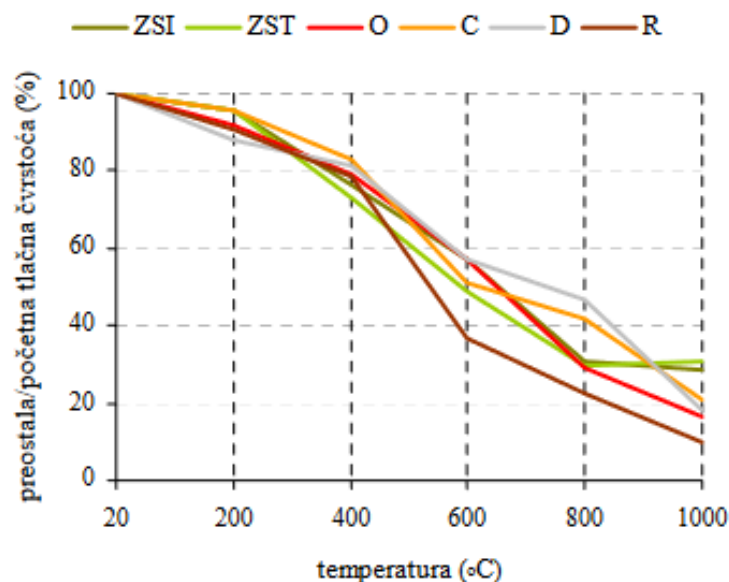
Slika 31. Odnos preostale i početne tlačne čvrstoće uzoraka s različitim agregatima nakon izloženosti visokim temperaturama [12]
