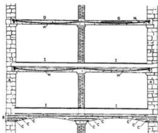
Slika 4. Betonski stropovi Wilkinsona [6]
