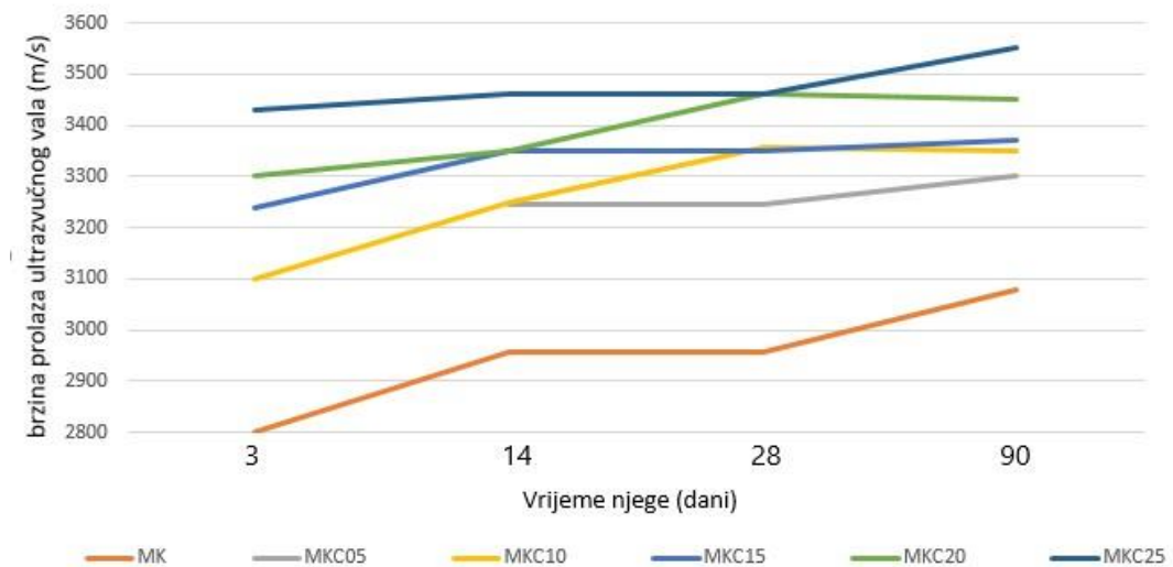
Slika 14. Brzina prolaska ultrazvučnog vala na uzorcima starosti 3, 14, 28 i 90 dana [12]
