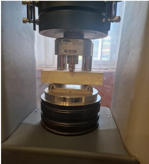
Slika 43. Ispitivanje vlačne čvrstoće
