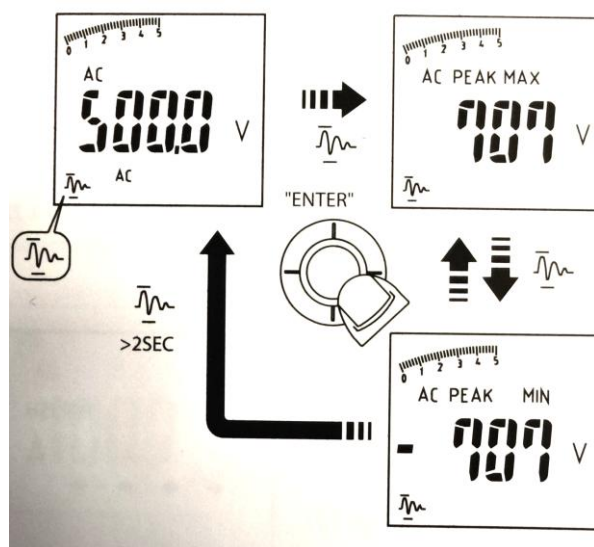
Slika 5.3 Peak Hold
