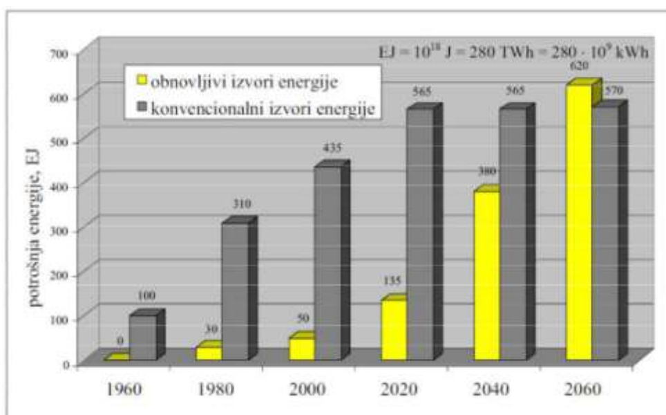
SLIKA 2.3. Plan rasta proizvodnje iz obnovljivih izvora energije i udio u ukupnoj potrošnji energije do 2060.godine [4]
