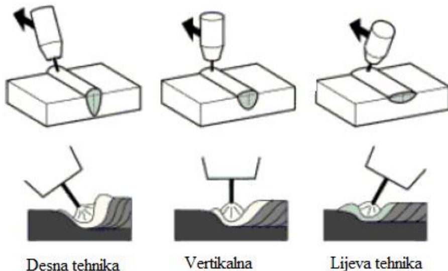
Slika 8.15 Vrste tehnika zavarivanja [18]
