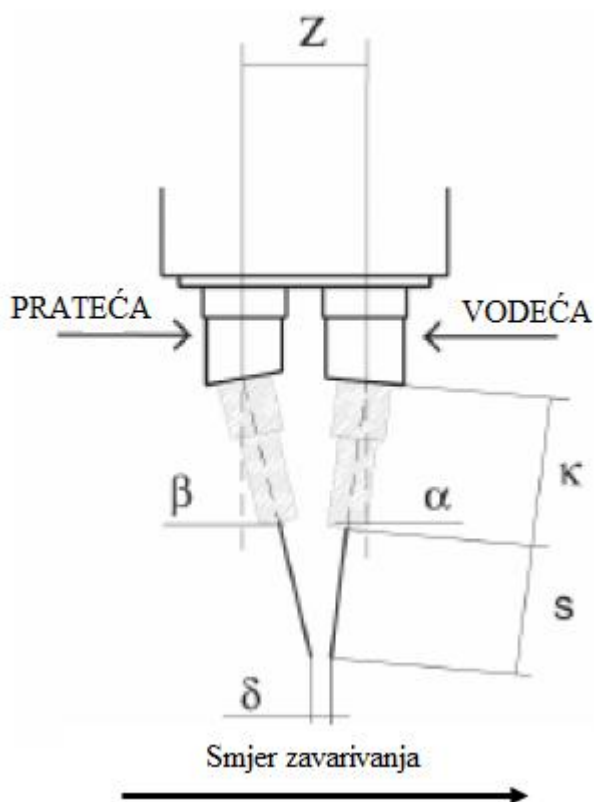
Slika 10.4 Definirana geometrija parametra pištolja [30]
