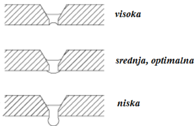
Slika 9.4 Utjecaj pozadinske struje na geometriju zavora [9]
