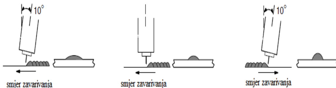
Slika 8.13 Nagib pištolja, utjecaj na oblik zavora [8]
