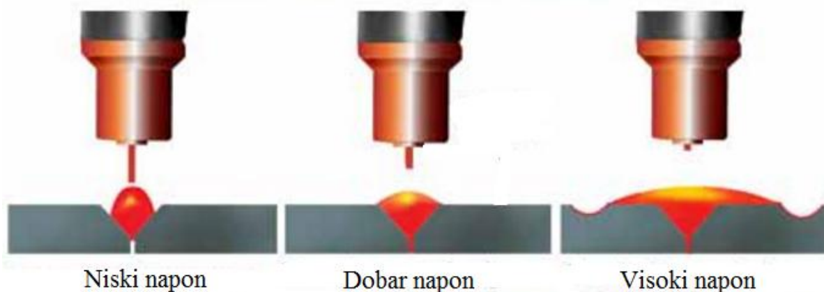
Slika 8.8 Shematski oblici zavora s obzirom na napon električnog luka [21]
