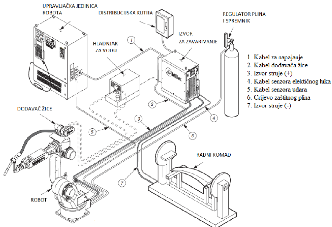
Slika 12.3 Robotska stanica [38]
