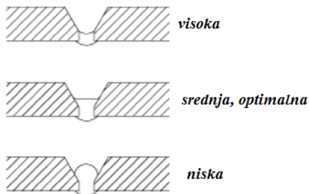
Slika 9.3 Utjecaj vršne struje na geometriju zavora [9]
