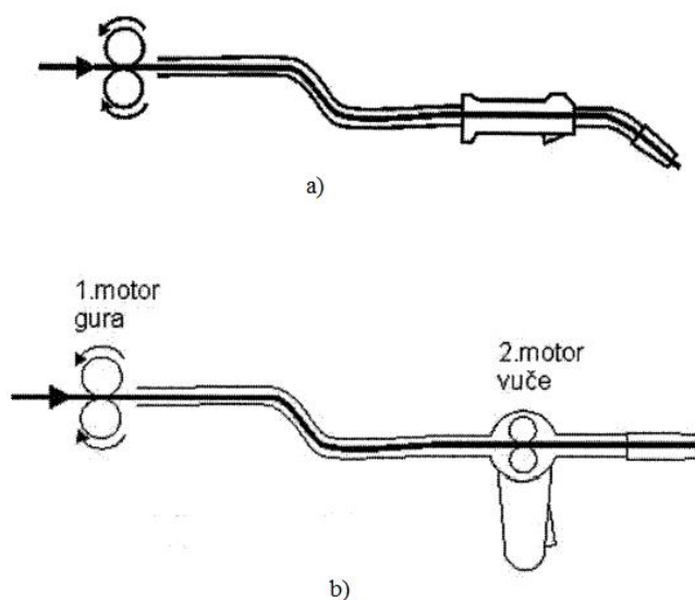
Slika 11.7 Dodavanje žice [31]
