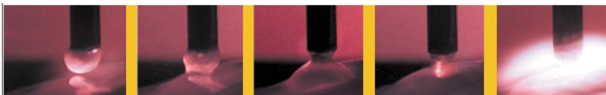
Slika 9.1 Slijed odvajanja kapljice kod STT postupka zavarivanja [23]
