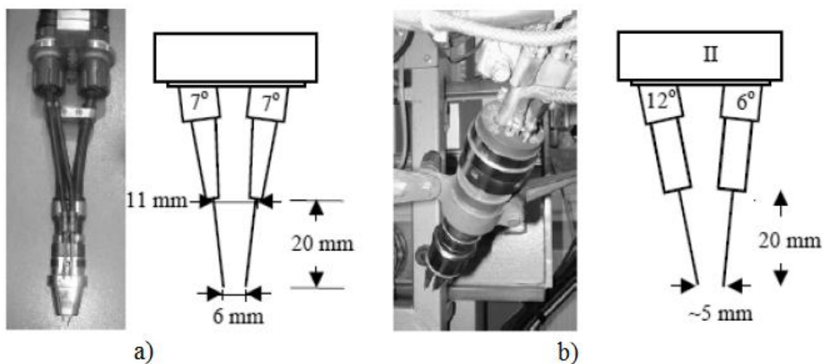
Slika 10.5 a) Closs pištolj sa fiksnim podešenim žicama, b) ESAB pištolj sa različitim podešenim žicama [30]
