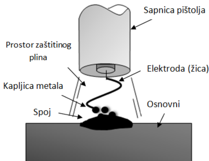
Slika 5.10 Shema prijenosa metala rotirajućim lukom [12]
