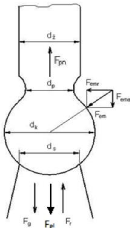
Slika 4.1 Shema sila [9]
