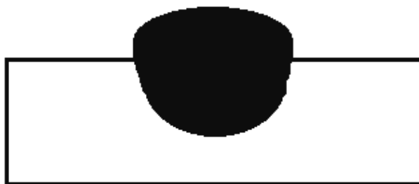
Slika 6.2 Utjecaj zaštitnog plina helija na geometriju zavora
