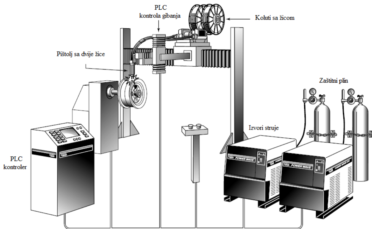
Slika 10.2 Tandem sistem [4]
