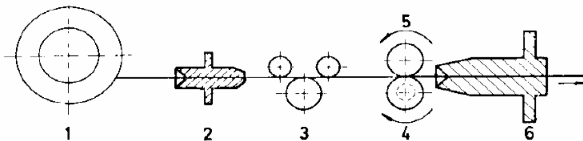
Slika 11.6 Shema dovođenja žice [5]
