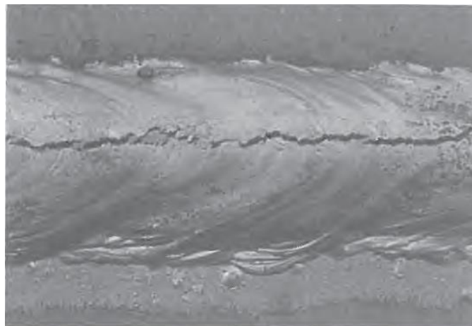
Slika 6. Karakteristična topla pukotina kod zavarivanja aluminija – sučioni spoj [1]
