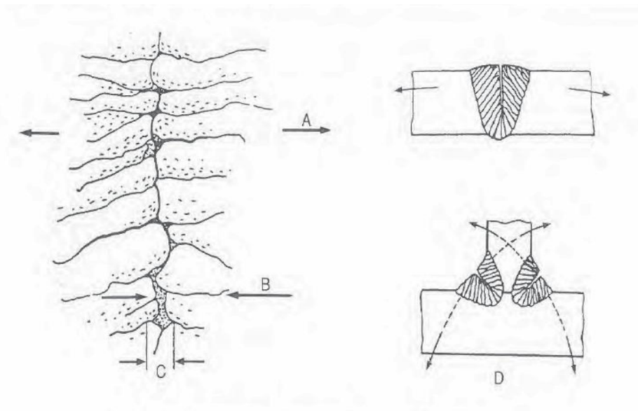
Slika 5. Shematski prikaz mehanizma nastajanja toplih pukotina [1]
