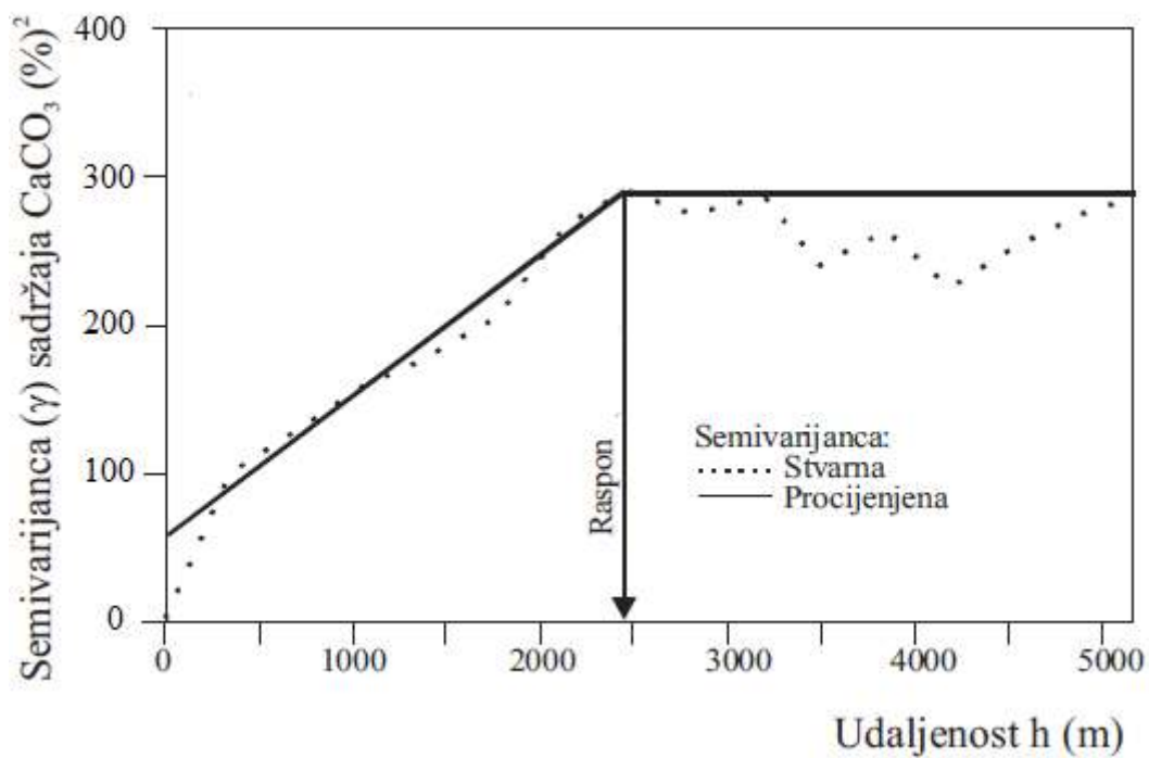
Slika 3.3.1 Eksperimentalni semivariogram sadržaja \text{CaCO}_3 iz dubine 0 – 30 cm
