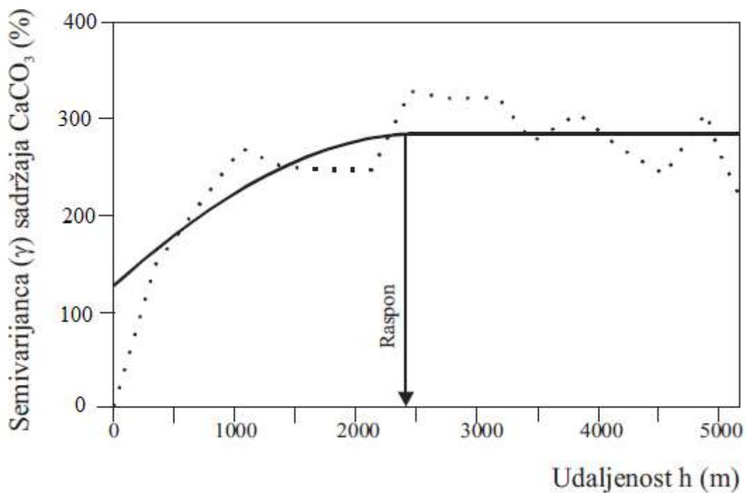
Slika 3.3.2 Eksperimentalni semivariogram sadržaja \text{CaCO}_3 iz dubine 30 – 60 cm
