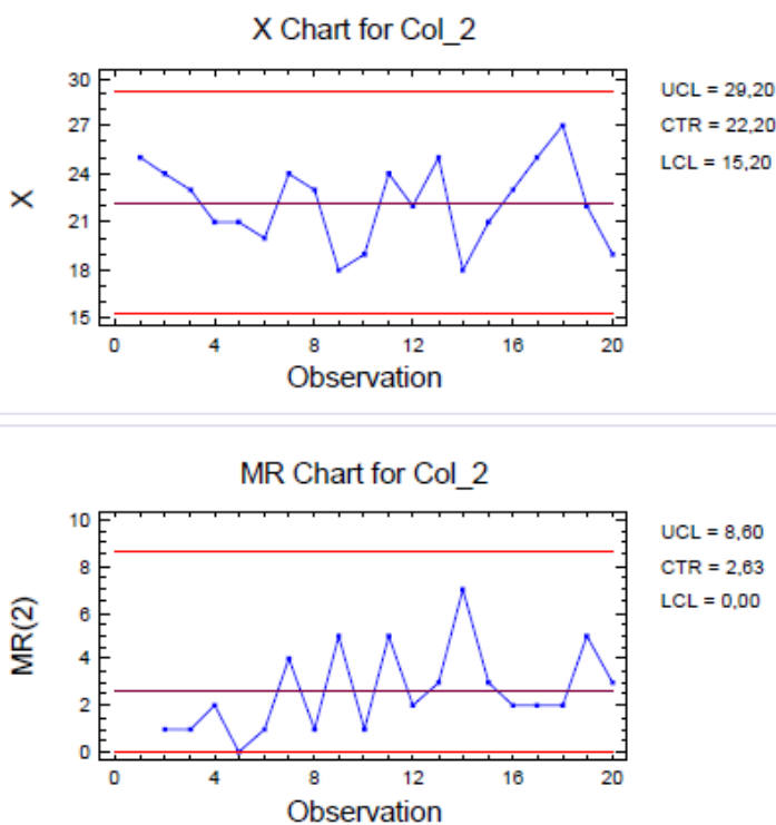
Slika 3.6: Primjer X-MR karte [5]
