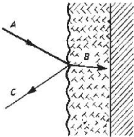
Slika 5.1.1. Apsorpcija zvuka u debelom poroznom sloju poroznog apsorbera
