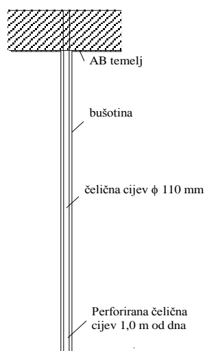
Slika 5.21. Skica temelj, bušotina, čelična cijev
