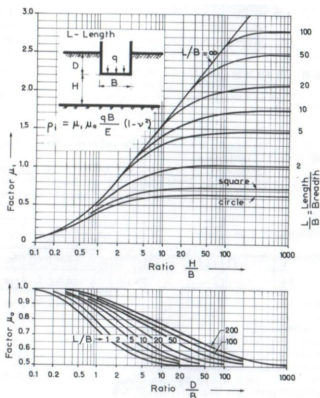
Slika 5.20. Bjerumovi dijagrami za faktore \mu_1 i \mu_0
