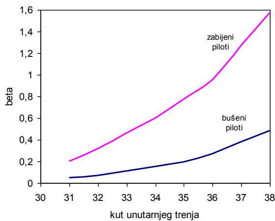
Slika 5.15.: Ovisnost \beta o kutu unutarnjeg trenja \varphi
