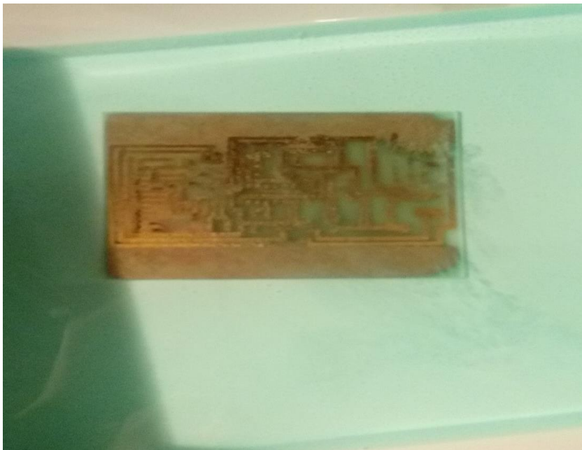
Slika 6.11. Jetkanje pločice
