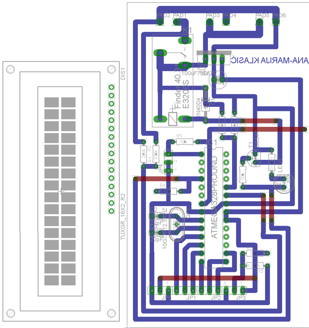
Slika 6.8. Raspored elemenata i vodova na tiskanoj pločici
